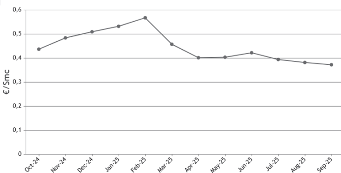
Grafico indice (12 mesi)
